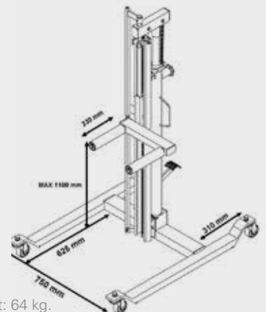
Fodbetjent løftefunktion.
